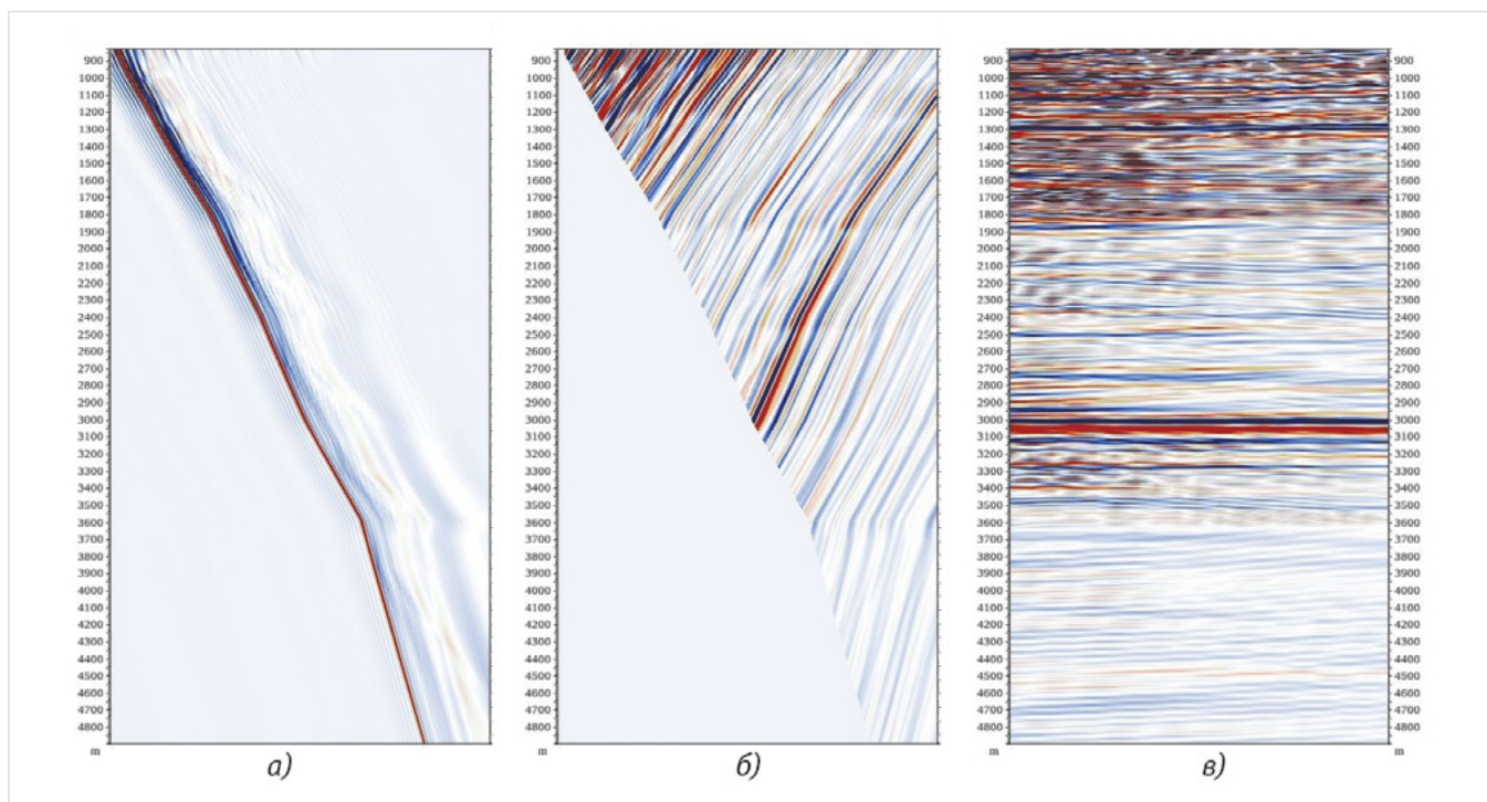
Рис. 1 — Пример данных способа псевдоВСП. Одно сечение трехмерной сейсмограммы на удалении источника от псевдоскважины на 600 м. Скважина в диапазоне глубин 830–4900 м, вынос скважины — 600 м, рассматриваемый диапазон времён — 530 м — 1750 мс, частоты — до 75 Hz, диапазон мигрированного разреза одного ОПВ +/- 250 м от скважины. А) прямая волна, рассчитанная в пластовой модели среды, в которой производилась послойная миграция. Б) Сечение трёхмерной сейсмограммы псевдоВСП. В) Фрагмент мигрированной сейсмограммы ОПВ в окрестности (+/-) 200 м от скважины
