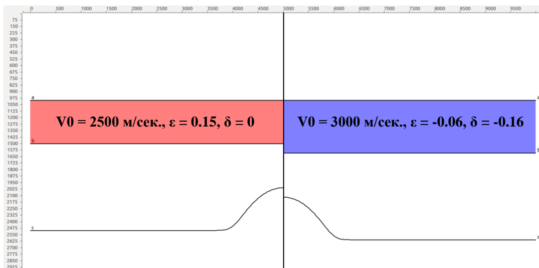
Рис. 1 Пример сечения двух совмещенных эквивалентных моделей. Левая половина изображает исходную модель, правая эквивалентную ей модель, полученную в результате решения обратной задачи определения оптимальных параметров анизотропии.
